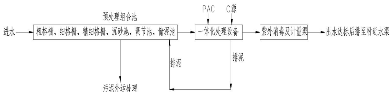
图3-4 污水处理厂运营工艺流程图
