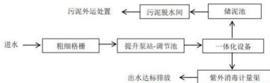
图 2-5 工艺流程图
