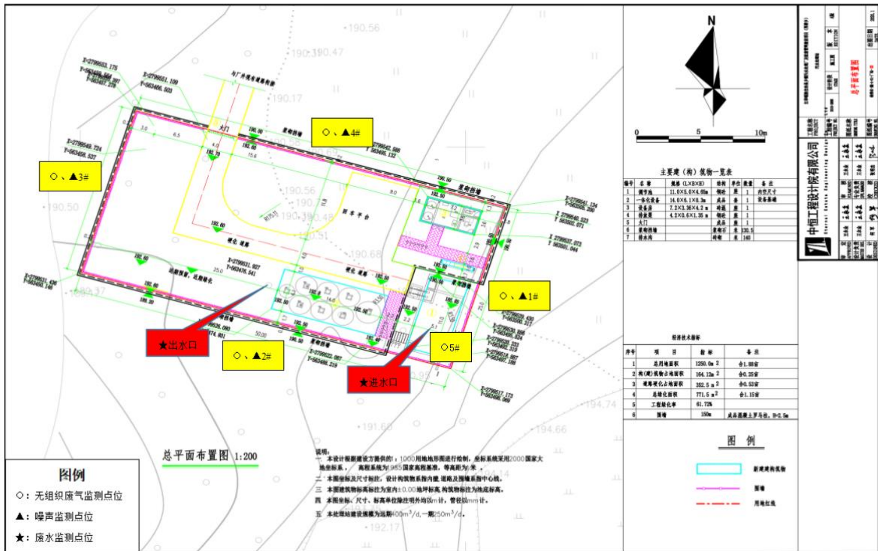
图3-3 平面布置图及监测点位图
