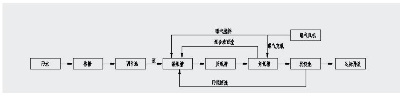
图3.3 污水处理厂运营工艺流程图
