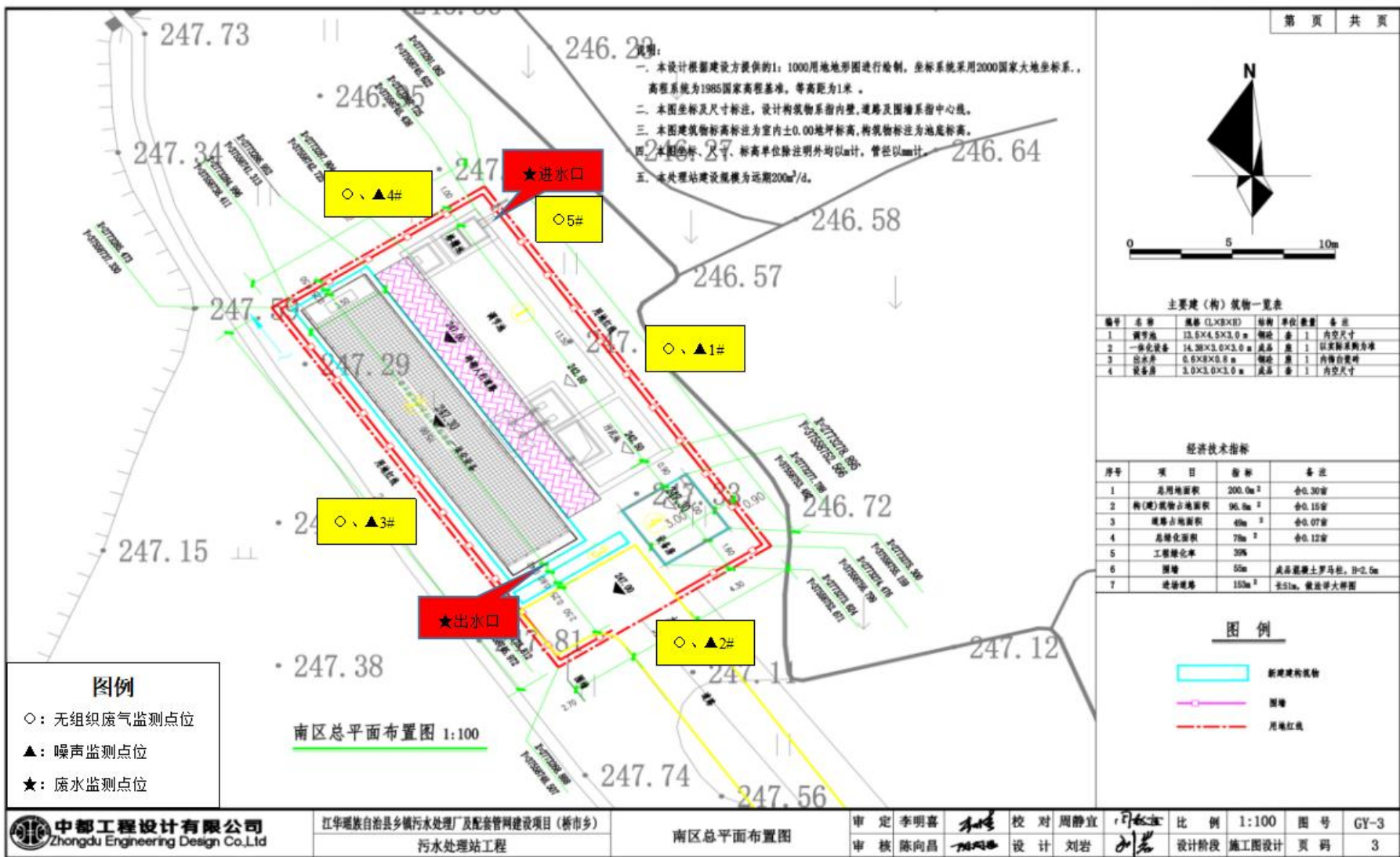
图3-2 平面布置图及监测点位图
