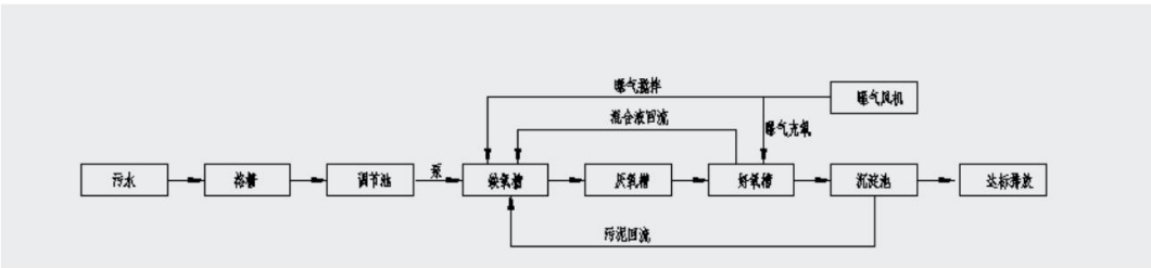
图 2-5 工艺流程图
