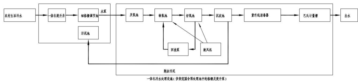
图 3.3 污水处理厂运营工艺流程图
