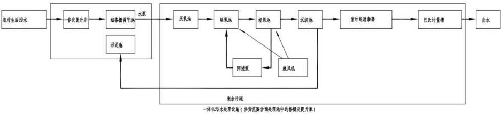
图 2.4-1 污水处理厂运营工艺流程图
