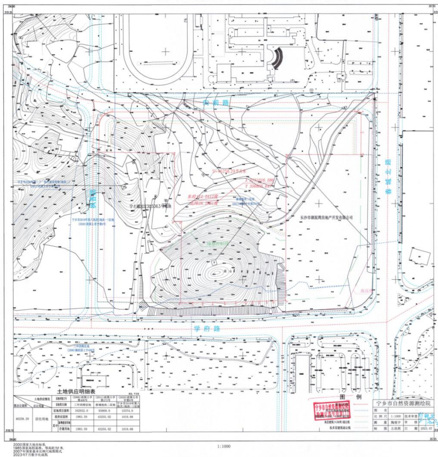
宁乡市土地储备中心202303064号拟出让地块图
