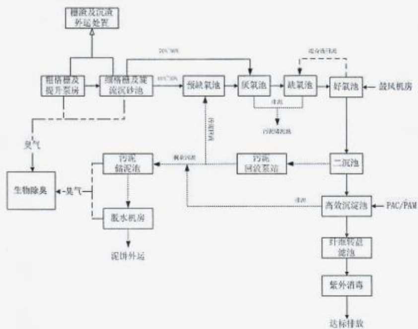
图 2.4-1 污水处理厂运营工艺流程图
